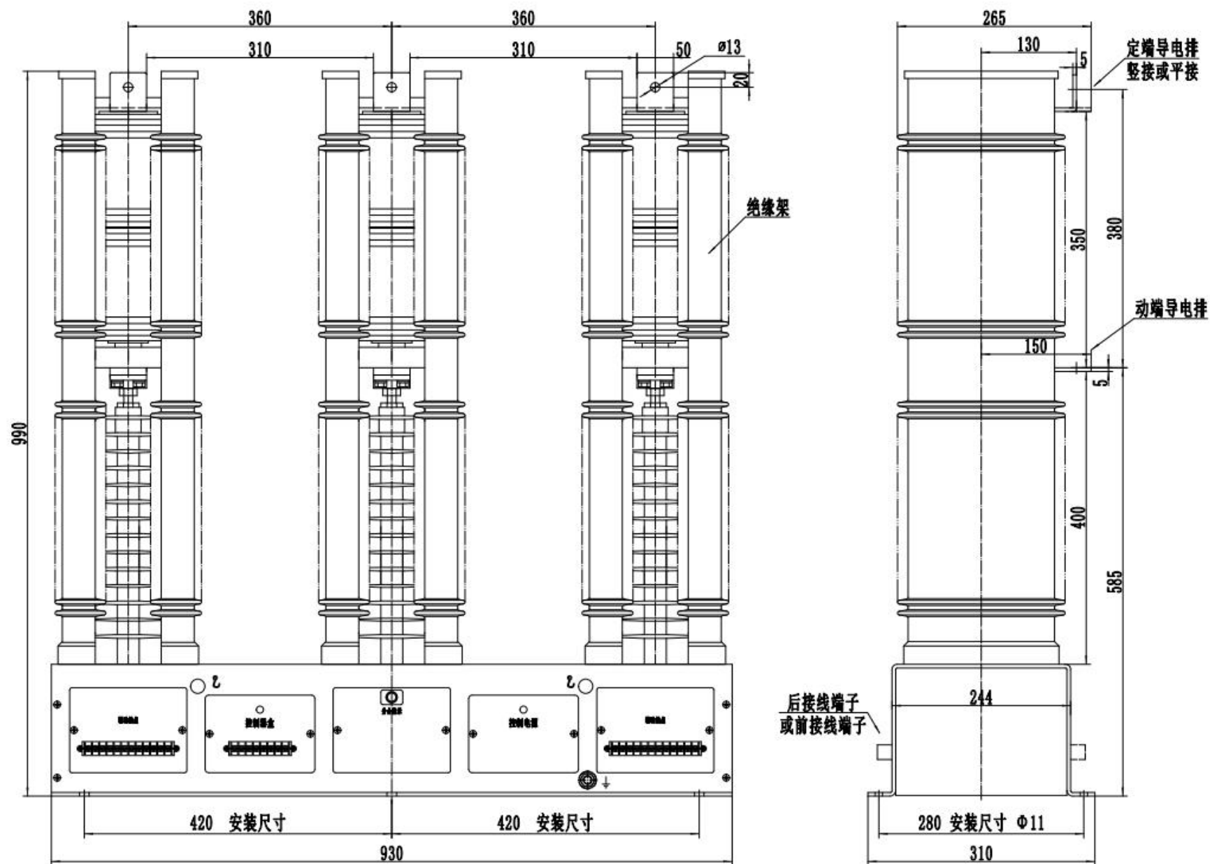
常规电磁机构外形及安装尺寸图
