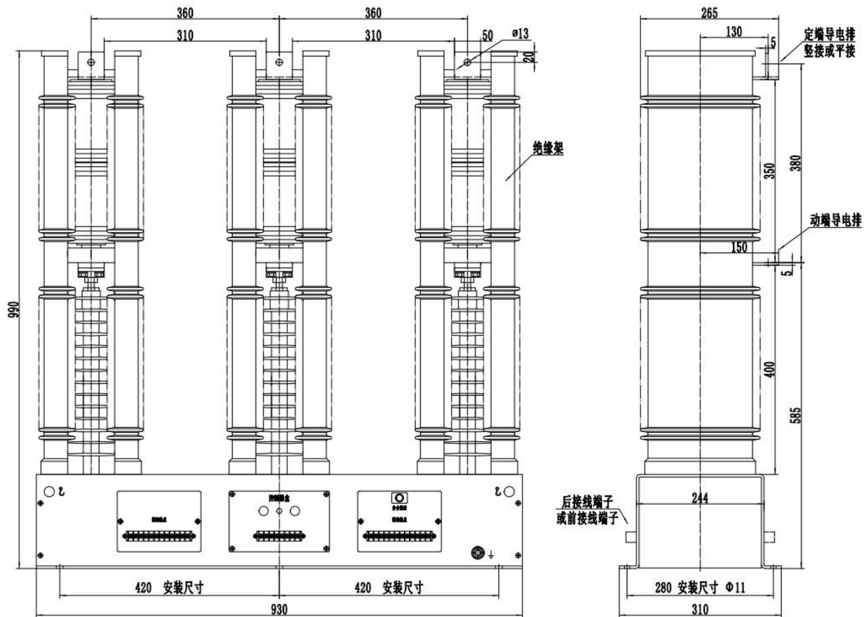
永磁机构外形及安装尺寸图
